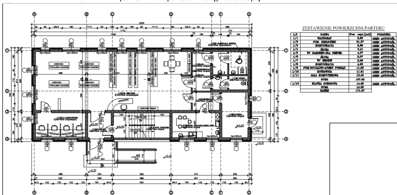
Rysunek 1 Rzut parteru – wstępna koncepcja
