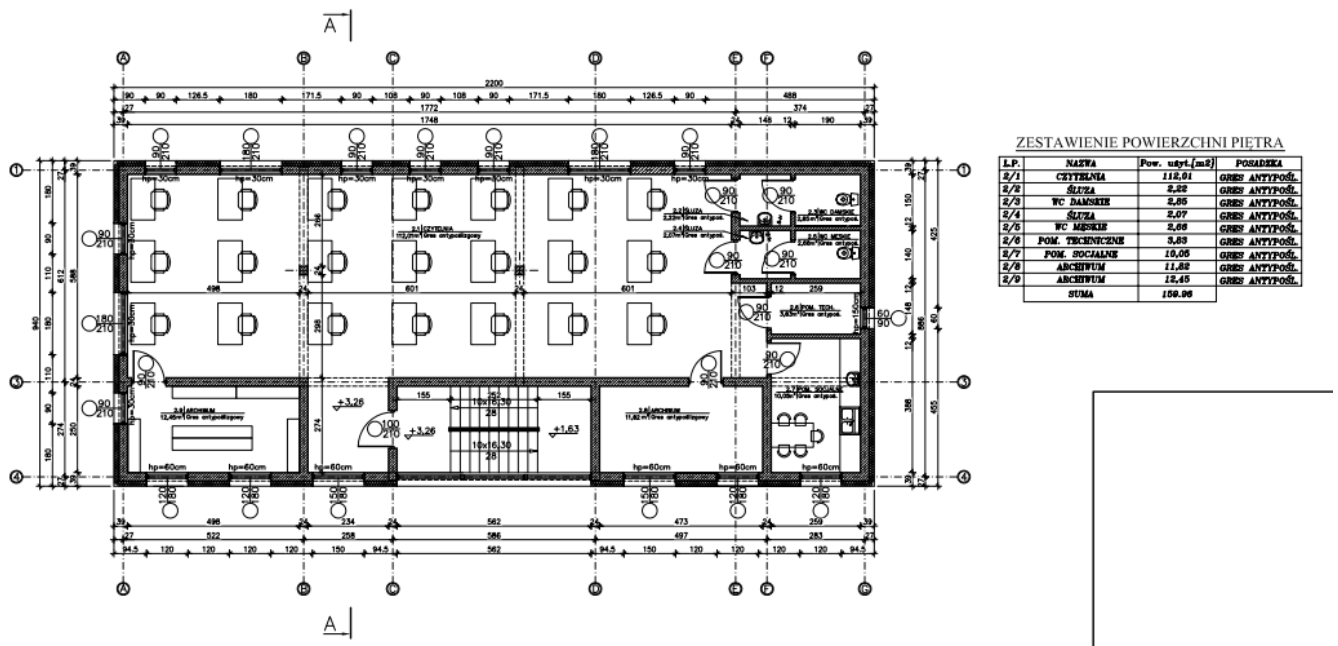
Rysunek 2 Rzut piętra – wstępna koncepcja
